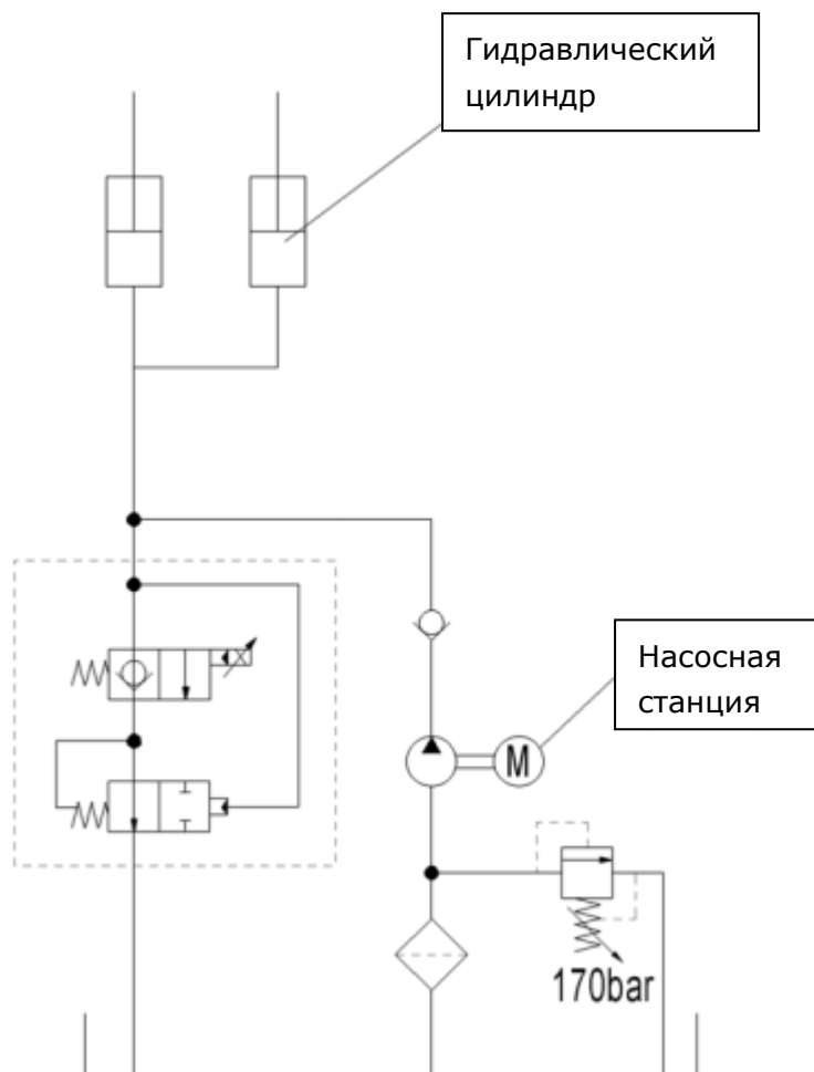
Рис. 26: Гидравлическая схема
