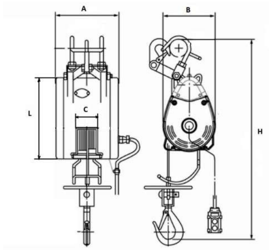
Рисунок 1. Размеры тали
