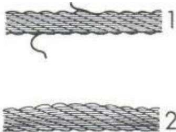
Проверка троса: (1) – использовать трос запрещено; (2) – трос готов к использованию.
