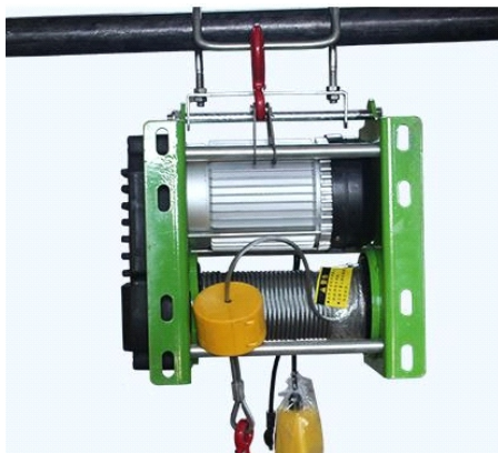
Рисунок 2. Крепление лебедки в вертикальном положении
