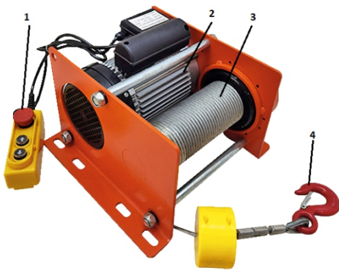
Рисунок 1. Конструкция лебедки
